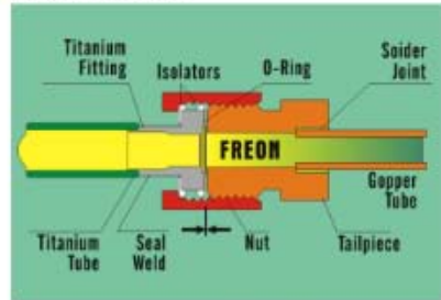
专利设计,电被彻底隔离,绝对安全
