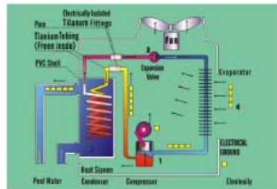
热泵工作示意图
